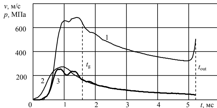
Рис. 4. Залежність швидкості истечения струи и давления внутри порохового ИВ от времени. 1 – скорость истечения, 2 – давление пороховых газов, 3 – давление воды в стволе, t_g = 1,57 мс – время горения пороха, t_{out} = 5,2 мс – окончание истечения струи воды.
