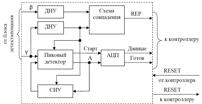
Рис. 2. Функциональная схема аналогового процессора
