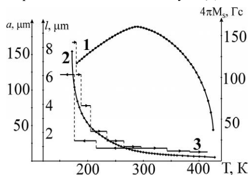
Рис.2 Температурные зависимости
