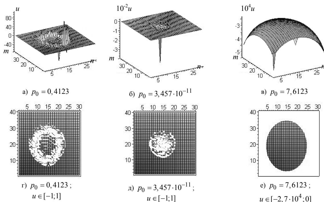
Рис. 2. Управление структурой поля деформации фрактальной эллиптической дислокации путем изменения параметра p_0 : зависимости функций смещения u (а, б, в) и их сечений (г, д, е) (вид сверху) от решеточных индексов n и m .
