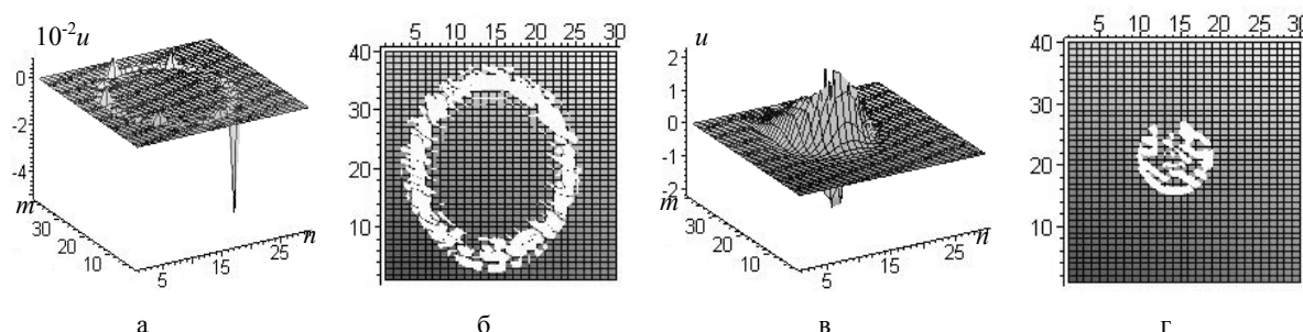
Рис. 1. Зависимости функций смещения u (а, в) и их сечений (б, г) при u \in [-1, 1] (вид сверху) от решеточных индексов n и m : а, б) для фрактальной эллиптической дислокации при p_0 = 1,0123 ; в, г) для фрактальной квантовой точки при p_0 = -0,2123 .
