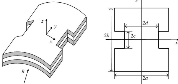
Рис. 1. Геометрическая форма и план оболочки
