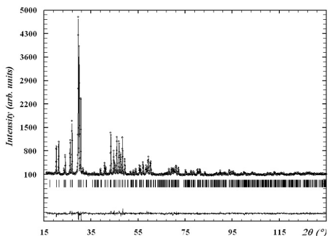
Рис. 1. Рентгенограмма Pb_8La_2(GeO_4)_4(VO_4)_2
