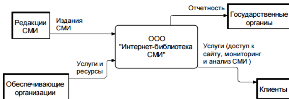
Рисунок 1.1 - Пример схемы взаимодействия с внешними контрагентами в DFD
